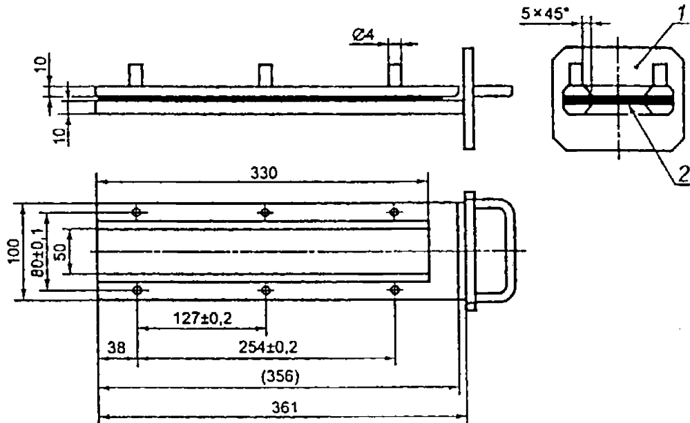
Рисунок 7.20 — Схема подставки
